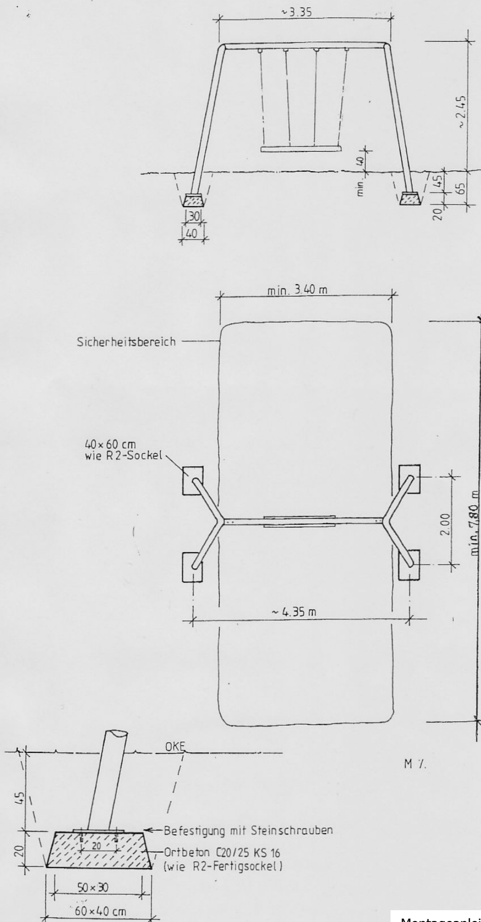
Montageanleitung 1.2.3. Schaukel aus Stahl 02 2931
